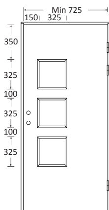
Type 15a
