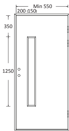
Type 18
