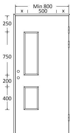
Type 13a
